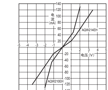
8. - (1) 输出部电流-电压特性 测定位置: 5-6端子间, 7-8端子间 环境温度: 25^{\circ}\text{C}
