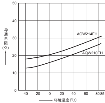
2. - (1) 导通电阻-环境温度特性 测定位置: 5-6端子间, 7-8端子间 LED电流: 5mA, 负载电压: Max. (DC) 连续负载电流: Max. (DC)
