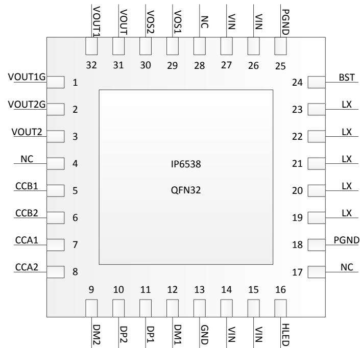
图 2 IP6538 引脚图
