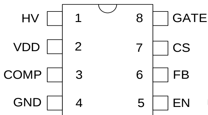
SOP8 封装
