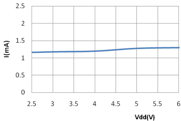
TA=20℃, Isopavg—Vdd 曲线
