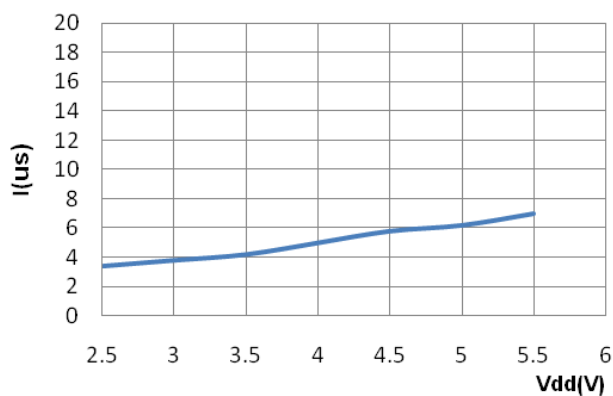
TA=20℃, Isstb—Vdd 曲线
