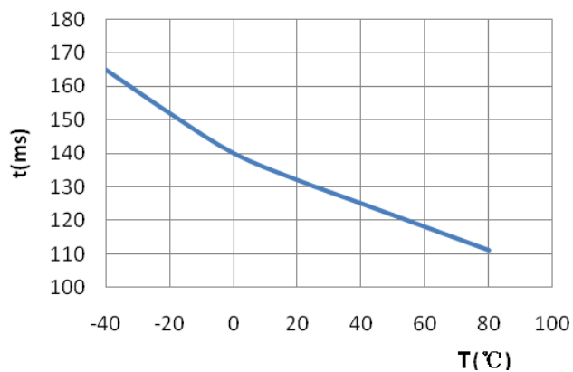
Vdd=2.7V, tstb—TA
