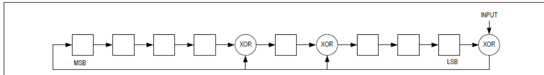
图 2-7 CRC 发生器
