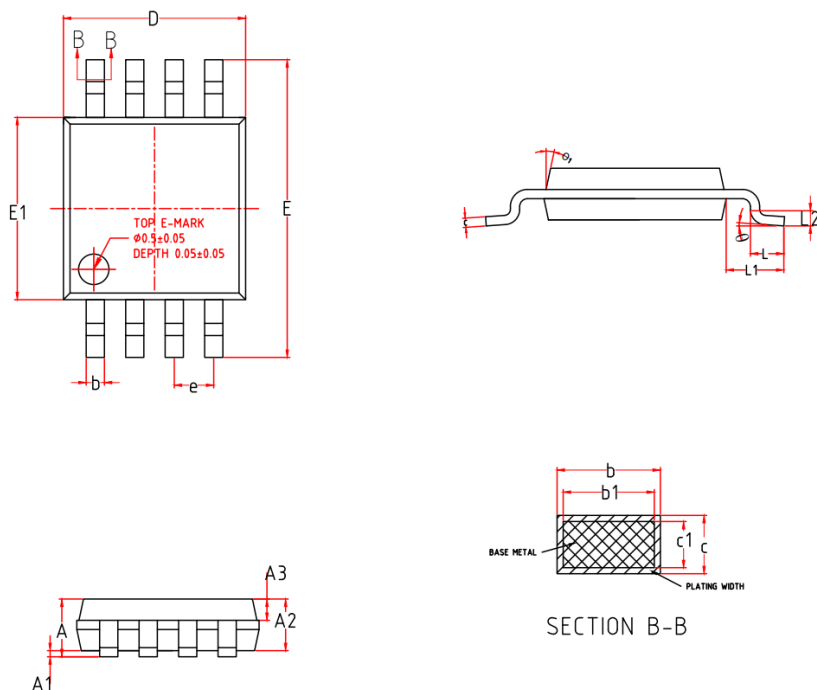
MSOP8 外形图
