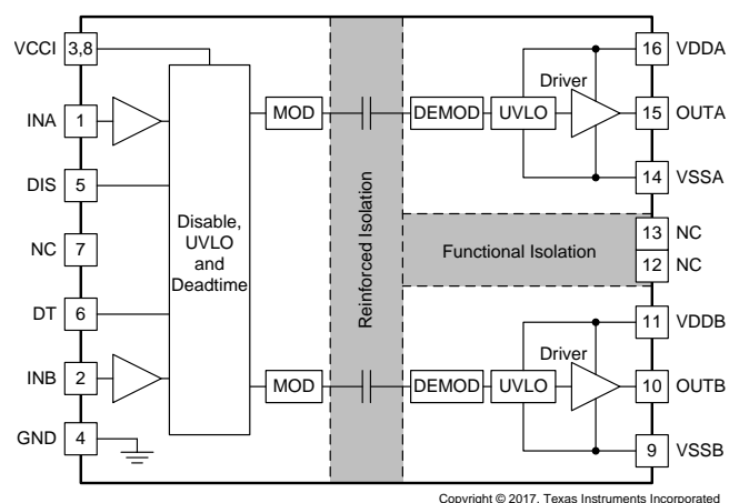
功能框图
