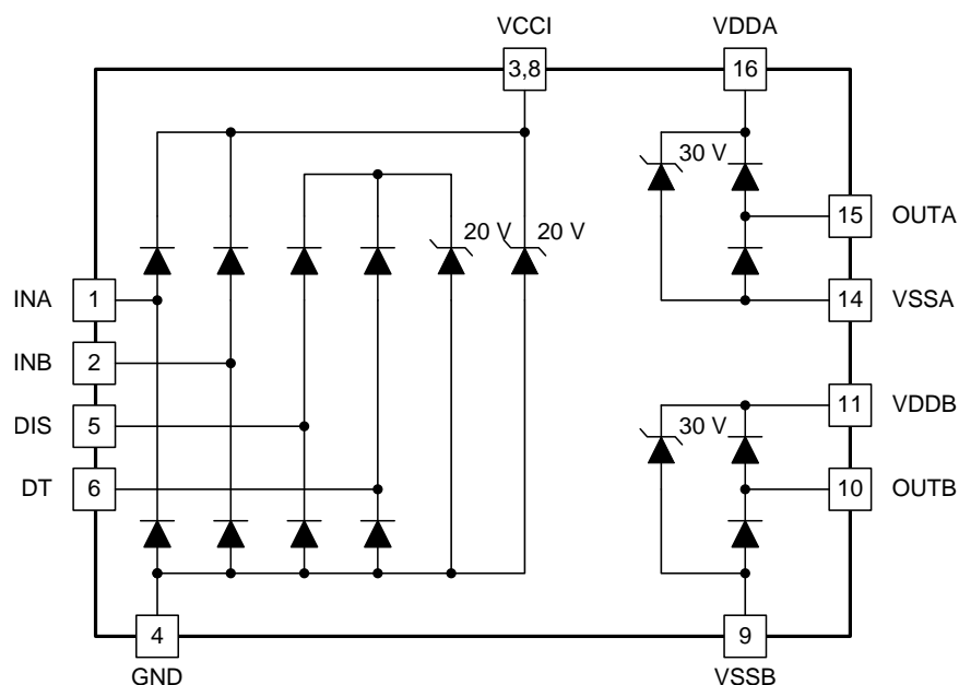
图 36. ESD Structure
