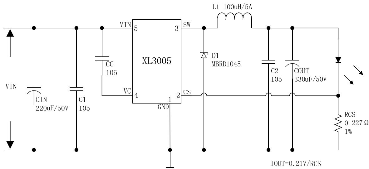
Figure17. XL3005 System Parameters Test Circuit (VIN=8V~36V, IOU=925mA)
