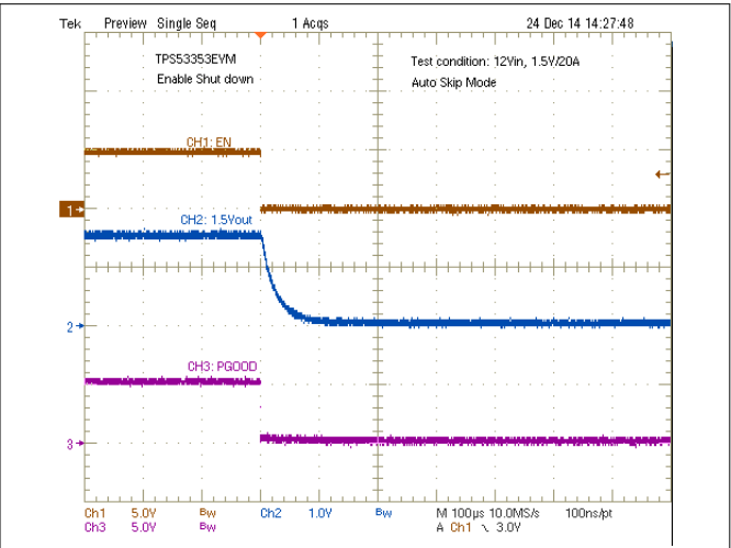
图 8-6. Enable Turnoff
