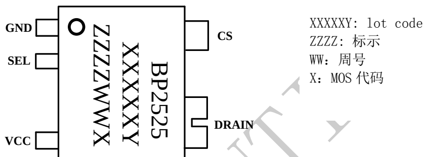
图 2 管脚封装图
