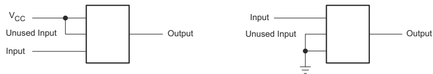
图 11-1. Layout Diagram
