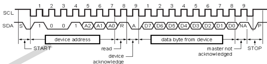
图 2-4 预置地址 1 字节（状态寄存器）读取命令
