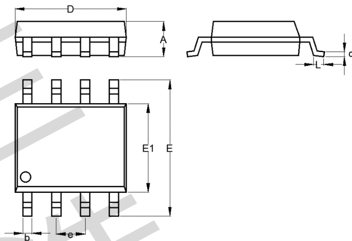
SOP8 外形图
