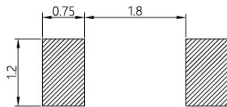
建议焊盘图
