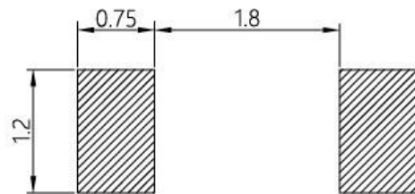
建议焊盘图
