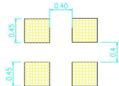
建议焊盘尺寸
