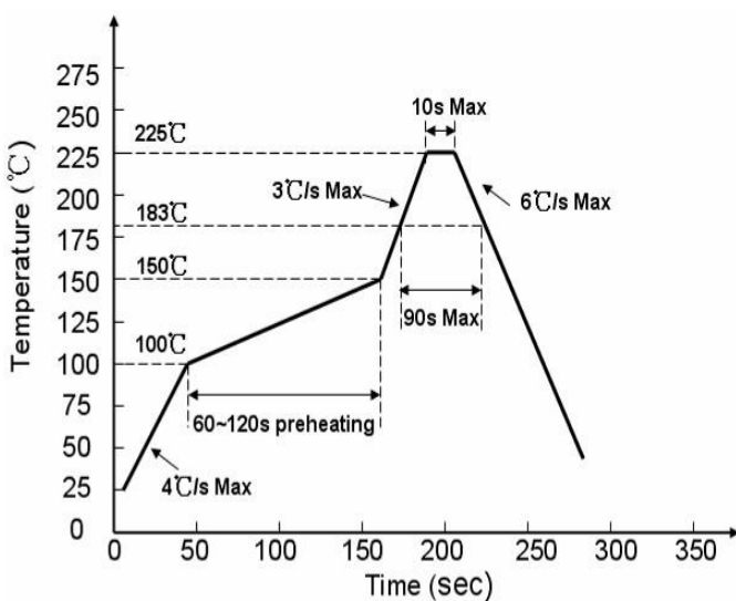
有铅制程
