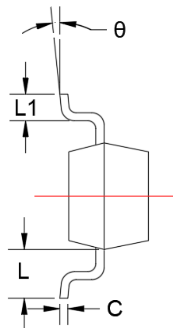
SOT-23
