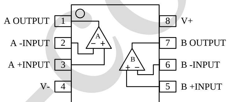
图 2 引脚图
