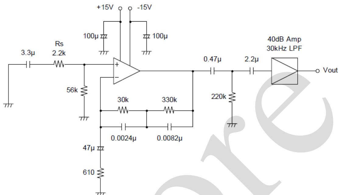
图 3 测试线路图
