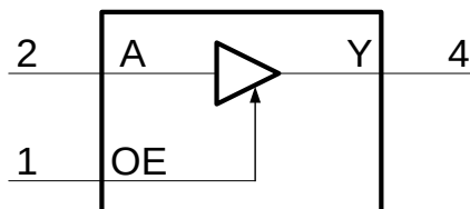
图 1 逻辑符号
