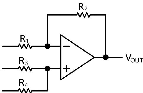
图 4. 差分放大器
