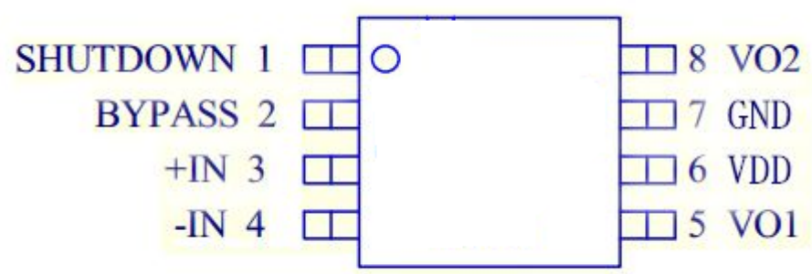
图 2. SD8002D SOP-8 封装管脚分布图
