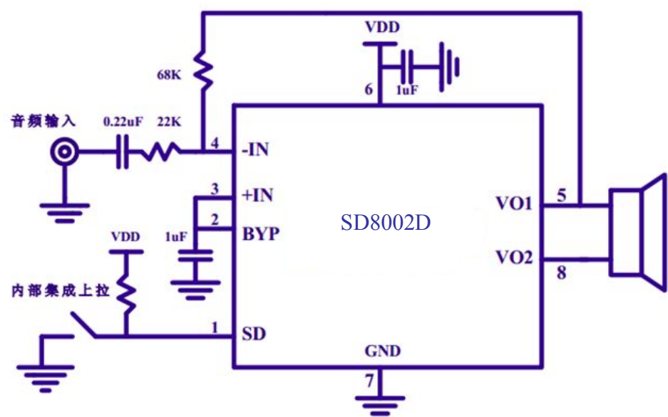
图 1. SD8002D 典型应用图
