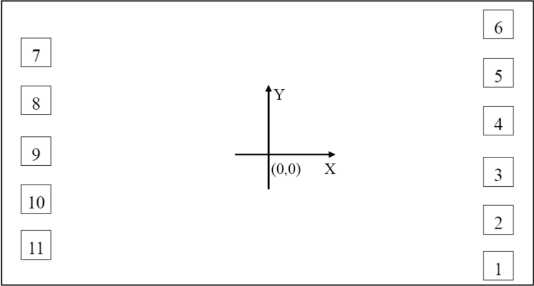
图 4 PAD 脚位图
