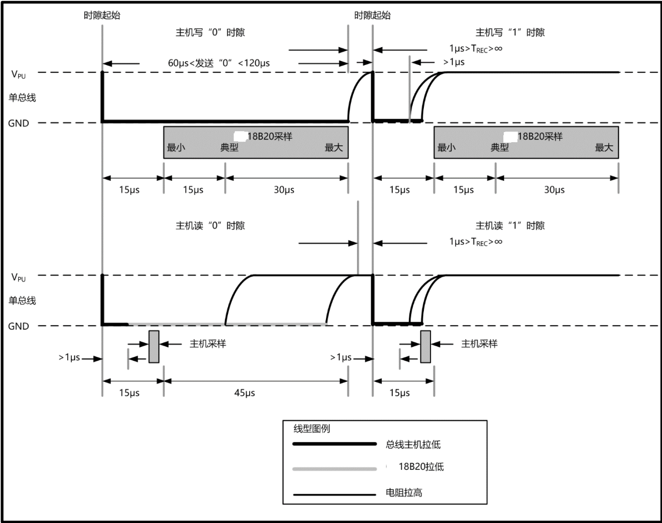
图 14 读/写时序
