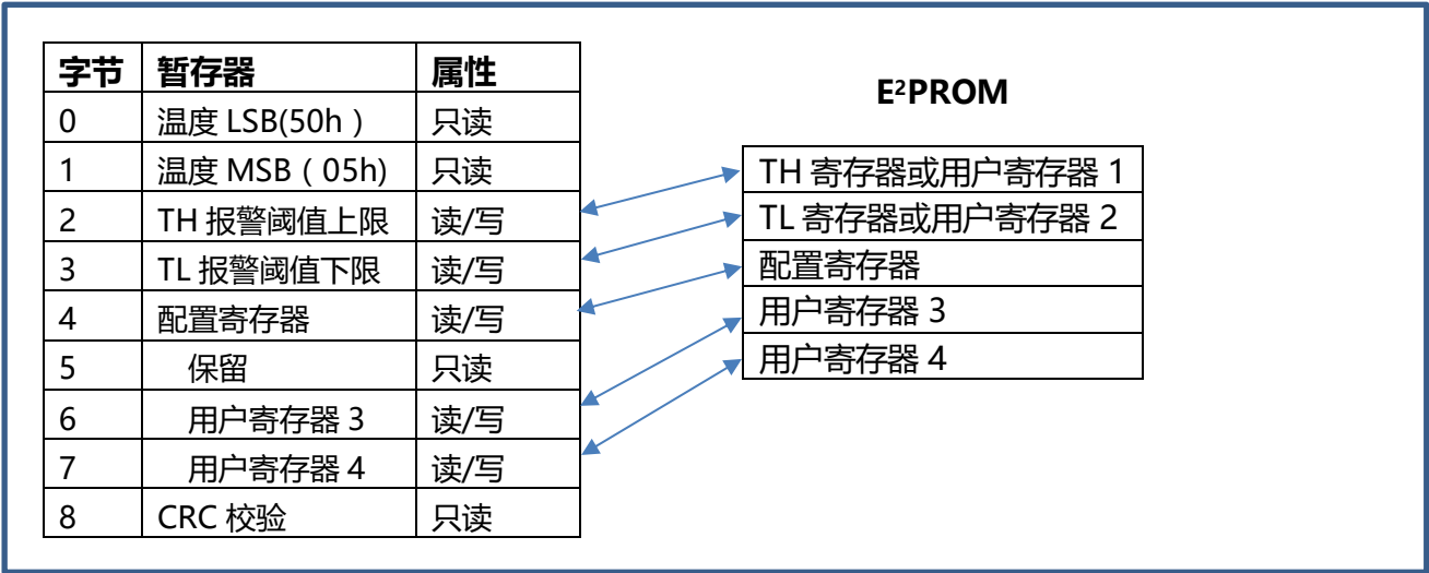
图 DS18B20 存储映射
