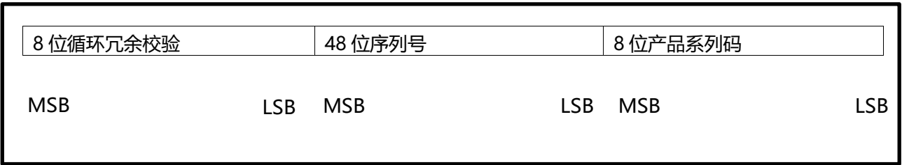
图 6 64 位激光 ROM 编码
