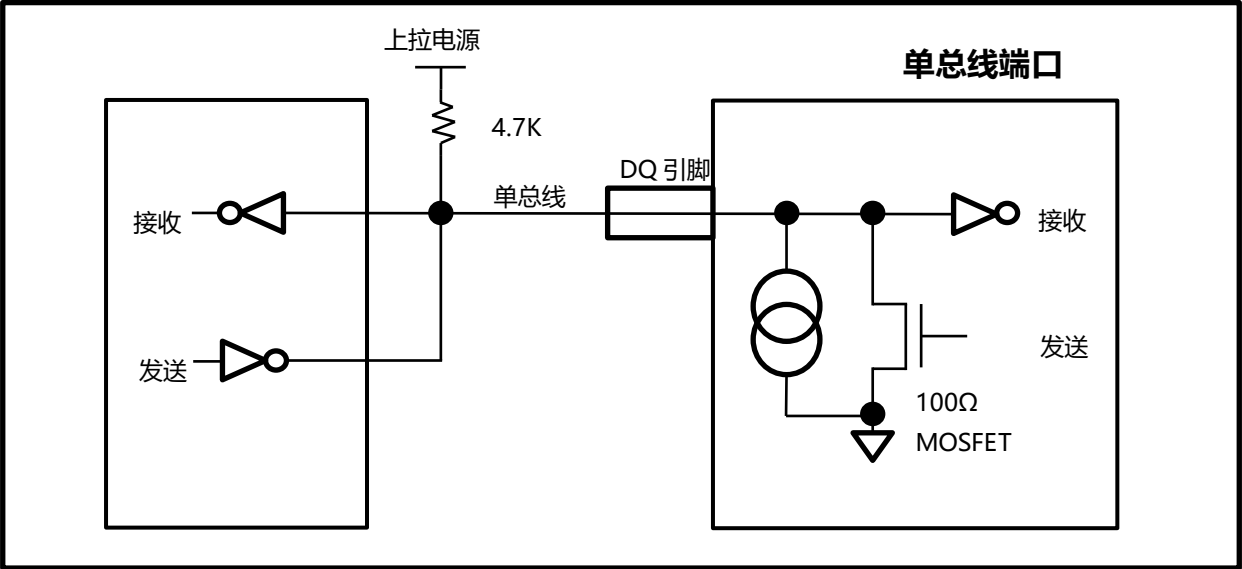
图 10 硬件配置
