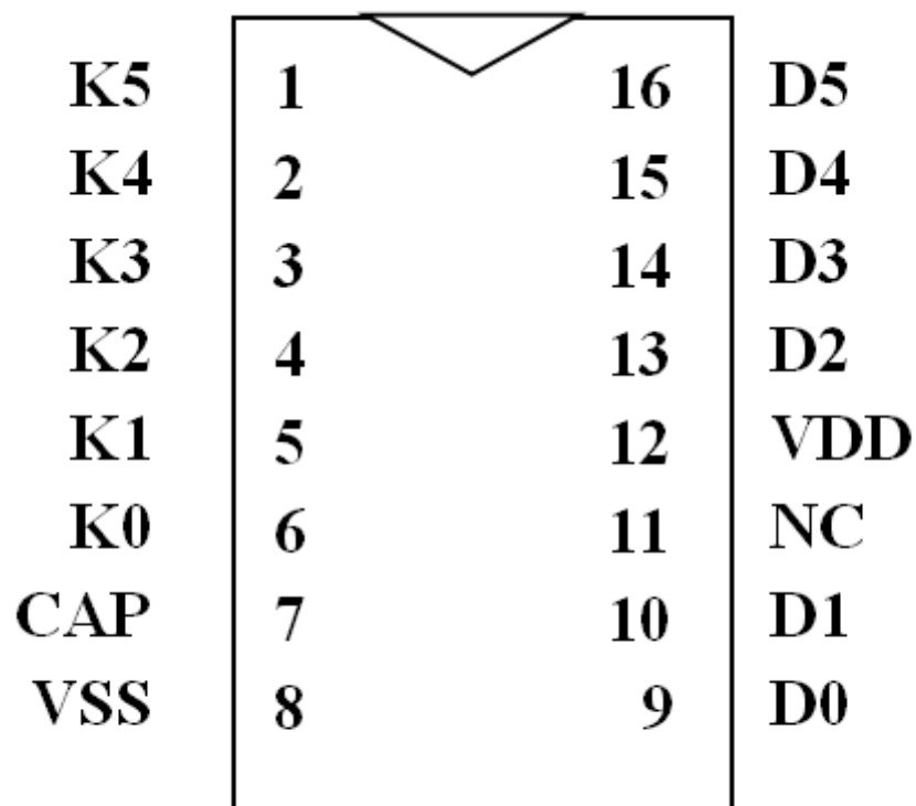
TTP272-AOBN 16-SOP-A
