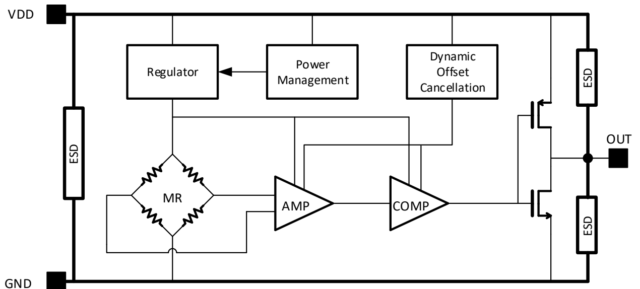
图 1 模块/线路图
