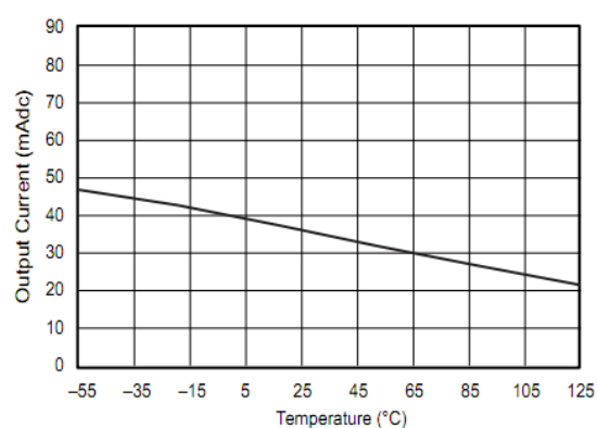
图 10: 输出拉电流限制
