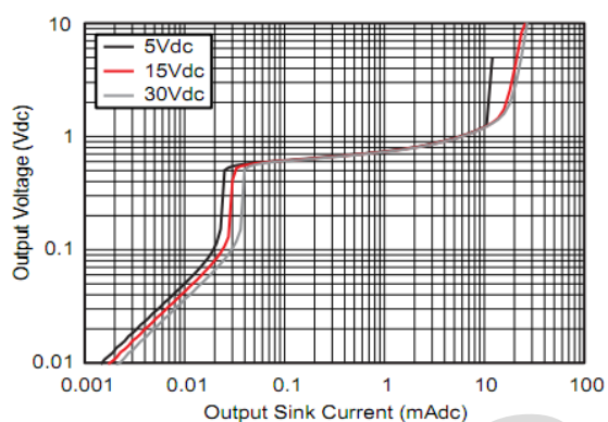
图 9: 输出灌电流
