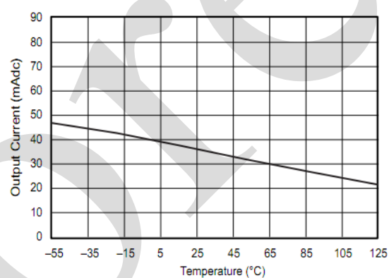
图 10: 源电流限制
