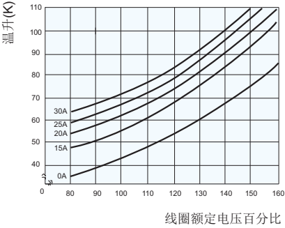
线圈温升
