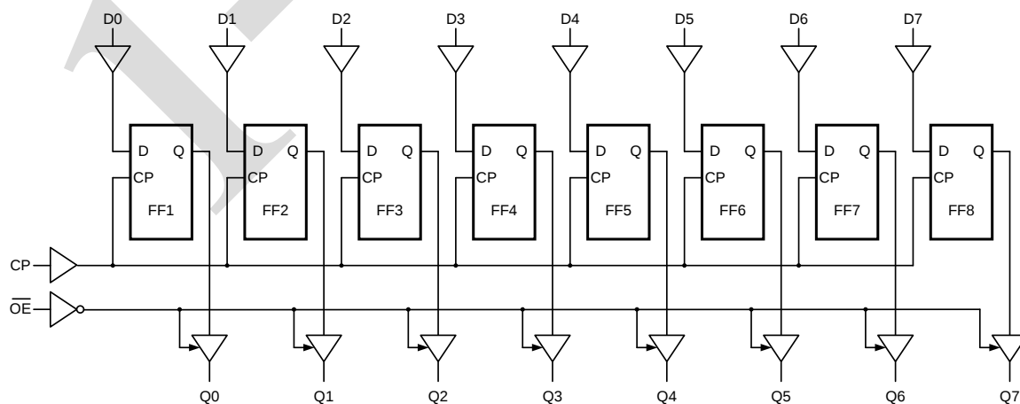
图 3 逻辑框图
