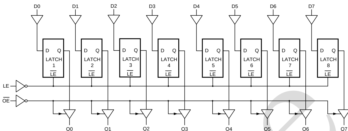
图 4 逻辑框图
