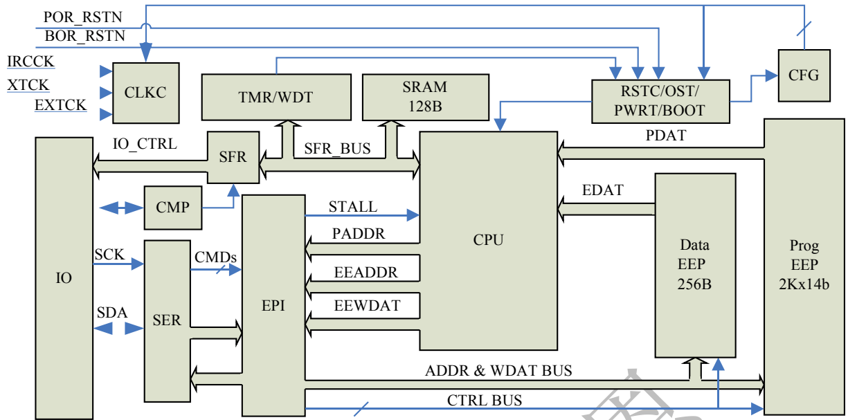
图 1.1 系统功能框图
