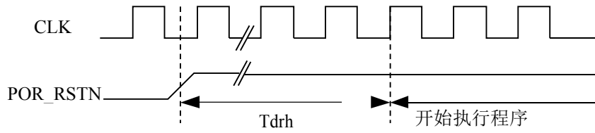
图 16.1 上电复位时序图
