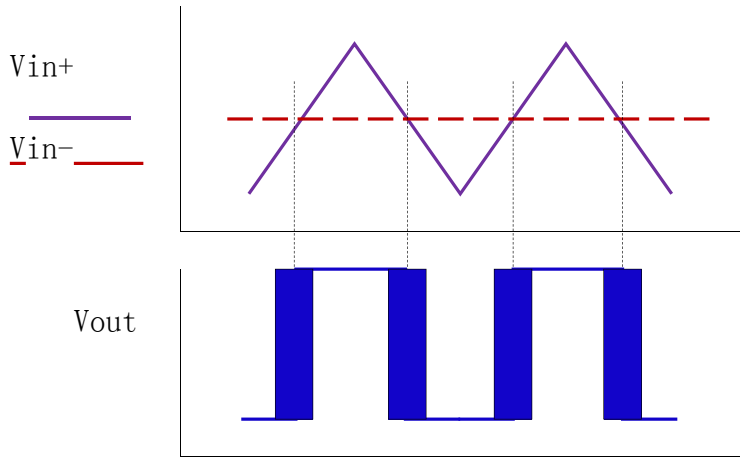
图 10.1 比较器的输入，输出信号特性 当比较器的输入和输出接近相等时，其输出为不定态，因此，为了避免这种不定态，或在某个输入端有微弱噪声存在，造成比较器输入出现不稳定态，一般比较器的设计会保护一个所谓迟滞电压，是 比较器的输出态变化会延后输入变化一定的距离，这样基本比较电平稍有波动也不会造成杂散输出信号。
