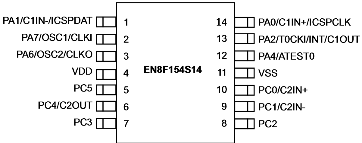
SOP14:EN8F154S14;DIP14:EN8F154P14;SSOP14:EN8F154SS14
