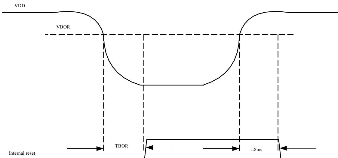
图 4.4 BOR 复位
