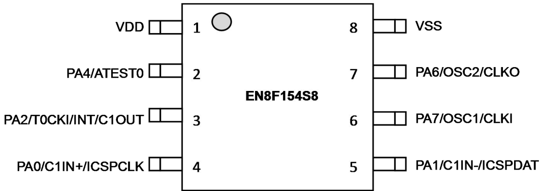
SOP8:EN8F154S8;DIP8:EN8F154P8
