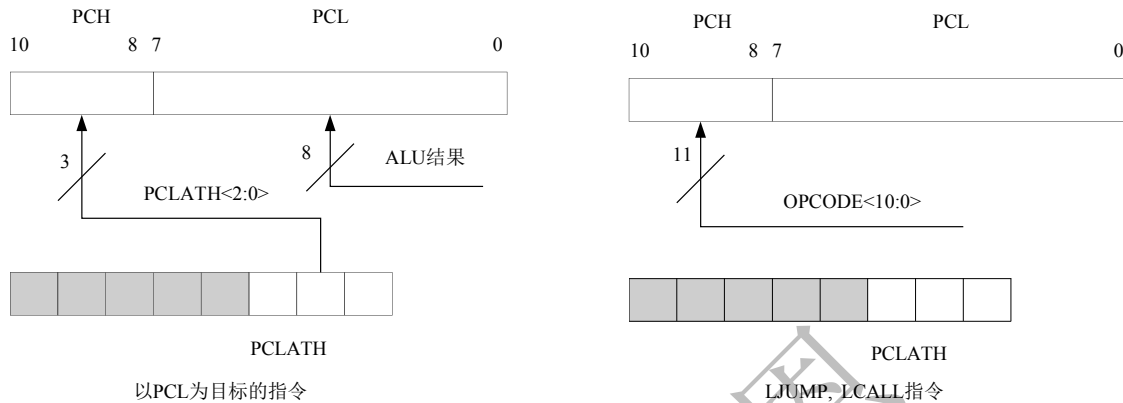
图 2.1.1 不同情况下 PC 的加载
