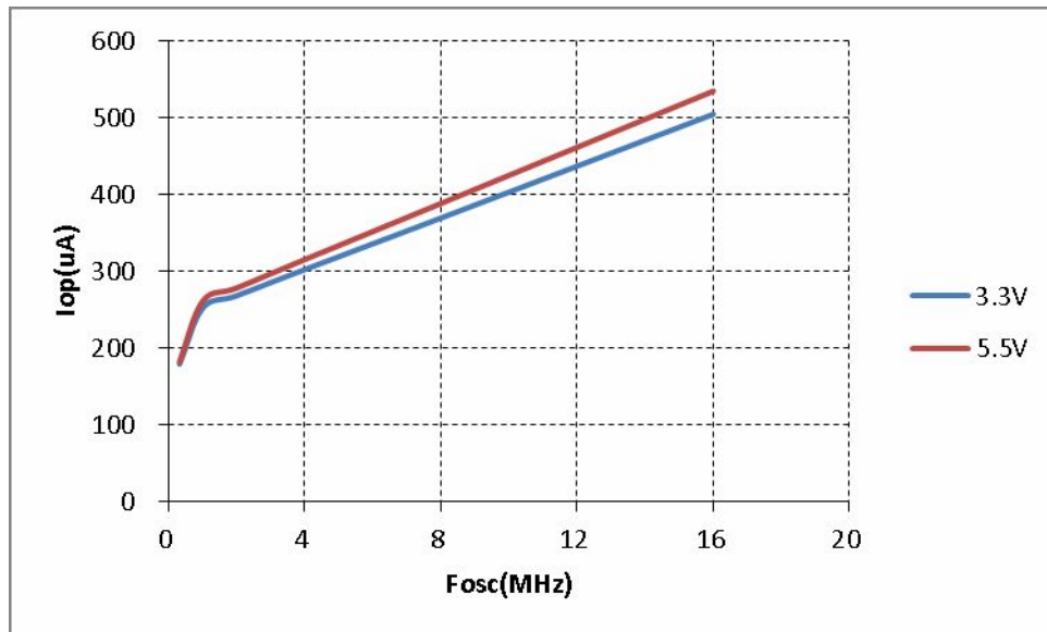
图 16.5 不同 VDD 下 Iop 与 Fosc 曲线 (T=25°C)
