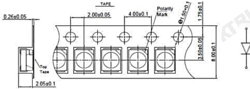
Tape Specifications (Units : mm) 载带规格 (单位: mm)
