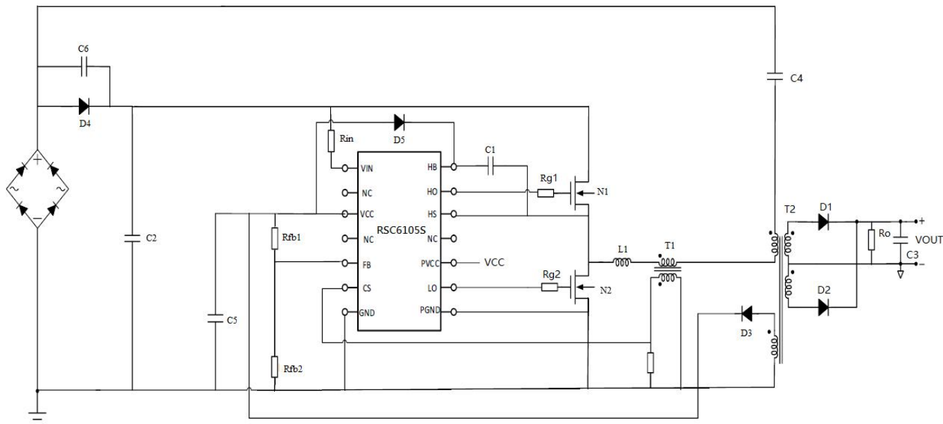
图 1: 典型应用图
