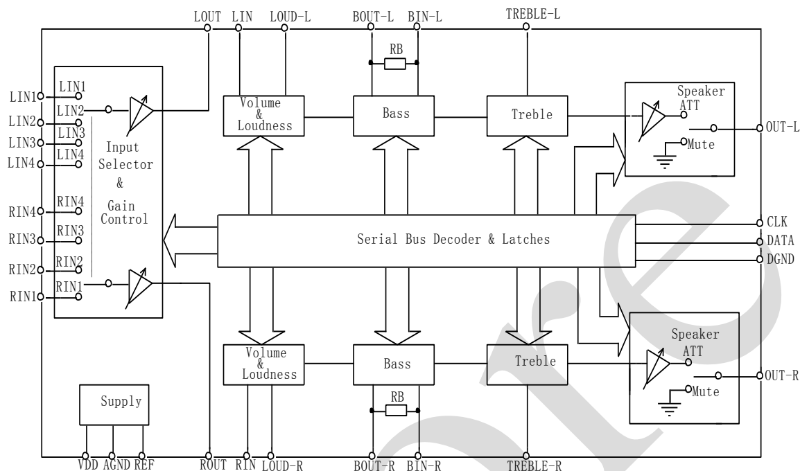
图 1、功能框图
