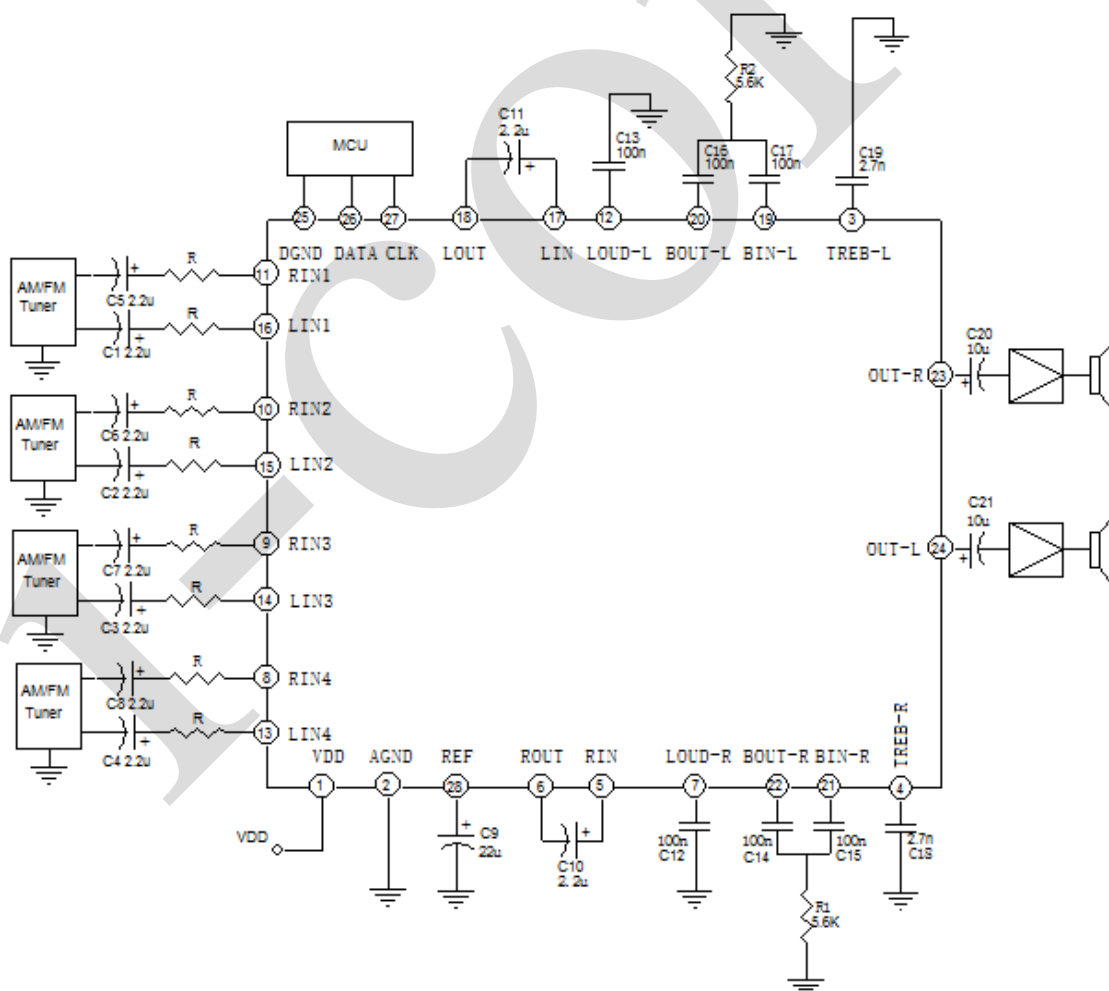
图 3、典型应用图
