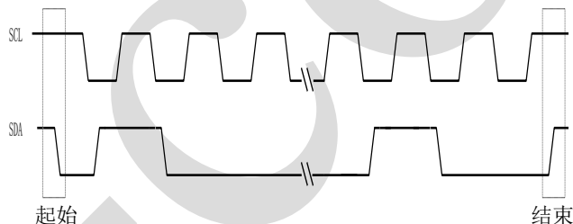
图 5、数据传输
