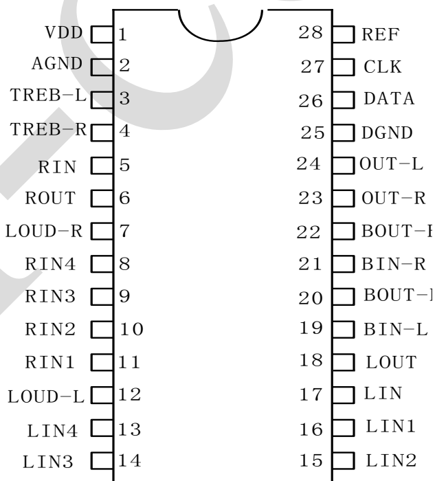
图 2、引脚排列
