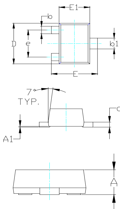
Package outline : SOT723
