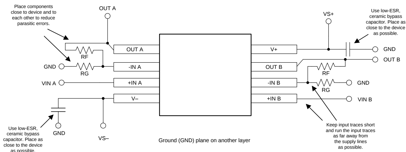
图 46. 布局示例
