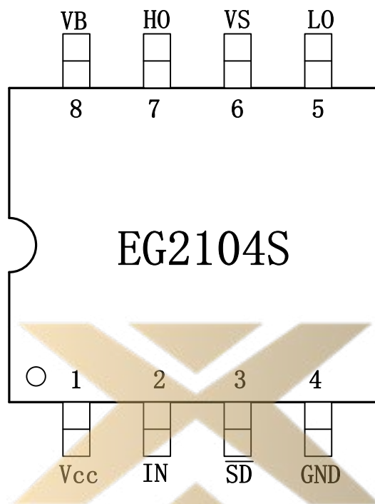
图 4-1. EG2104S 管脚定义
