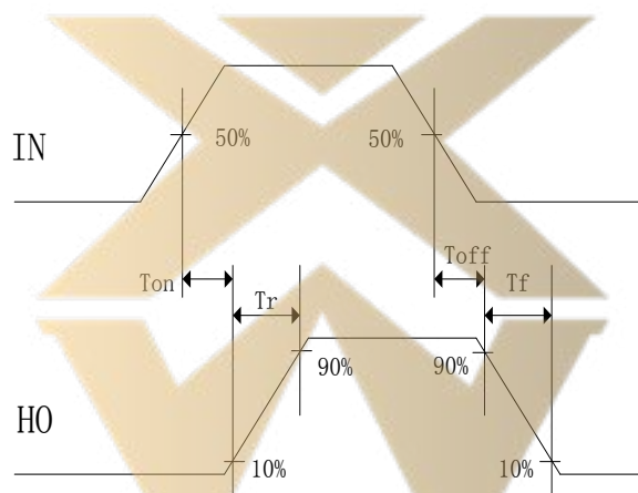
图 7-2. 高端输出 HO 开关时间波形图
