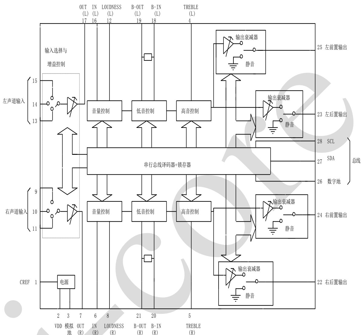
图 1、功能框图
