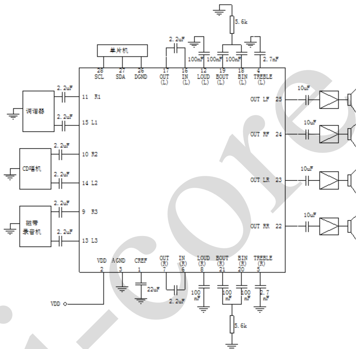
图 3、典型应用图
