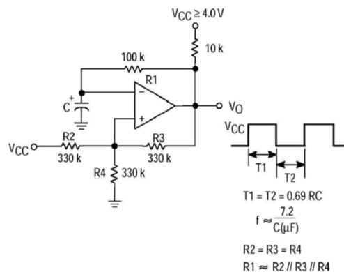
方波振荡器
