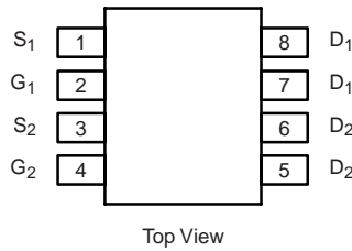
SO-8
