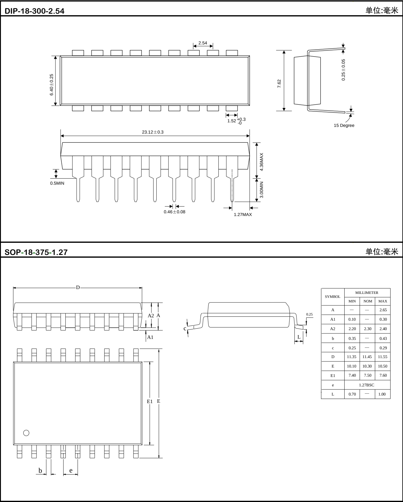
封装外形图
