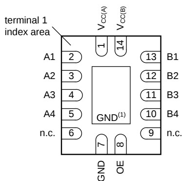
DHVQFN14
