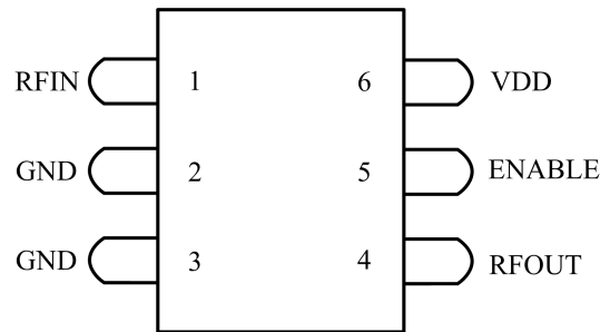
图 2-1 芯片封装管脚排列
