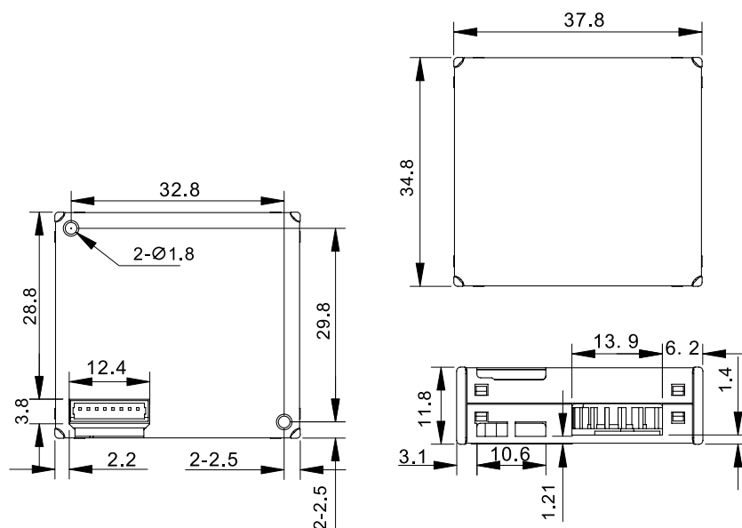
MPM10-AS 单位: mm
