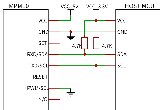
IIC 接口的电路连接
