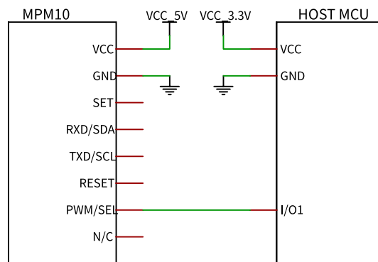
PWM 输出的电路连接
