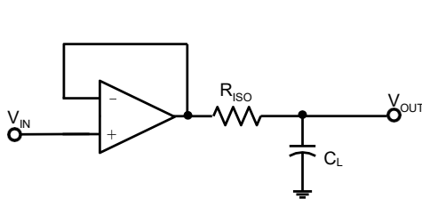
图3 驱动电容负载电路
