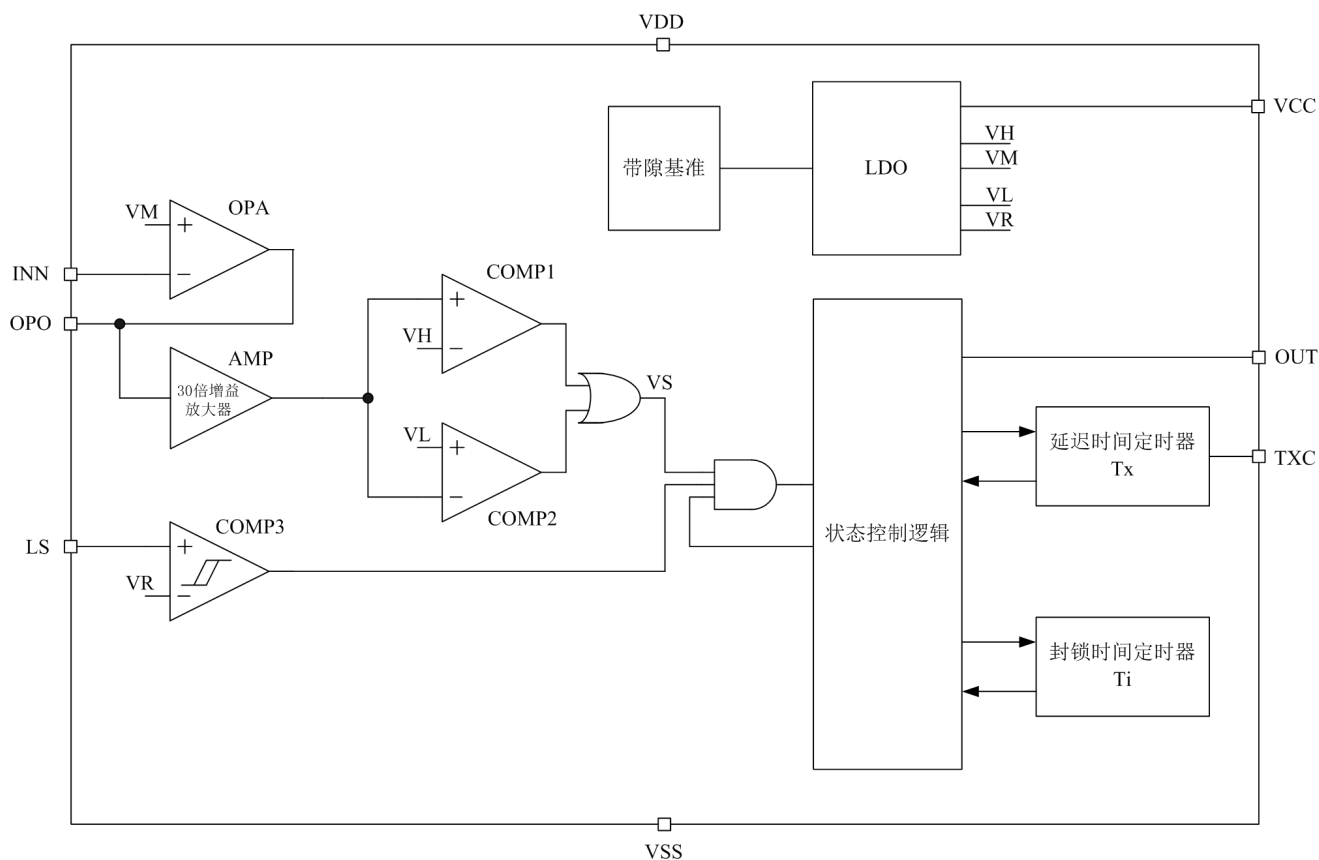
图 2: RS012 的内部电路方框图
