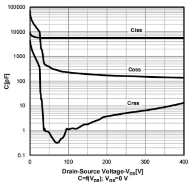
Typ. capacitances
