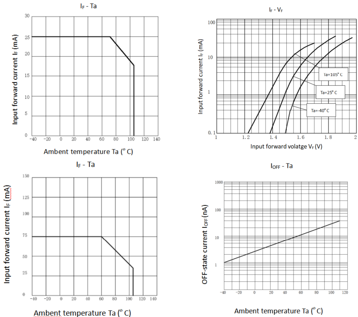
图 3 特性曲线
