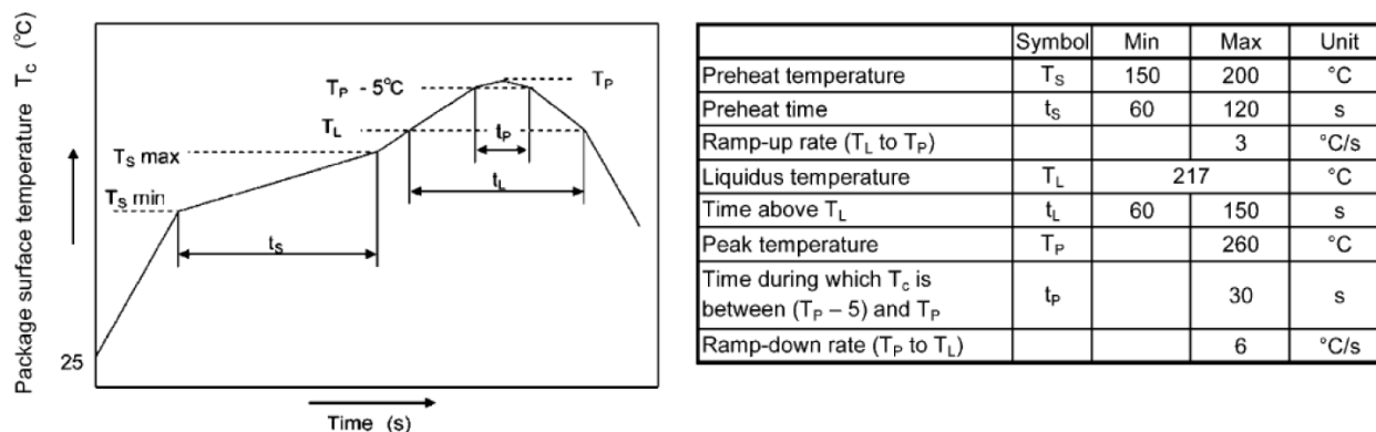
图 8 回流焊参数
