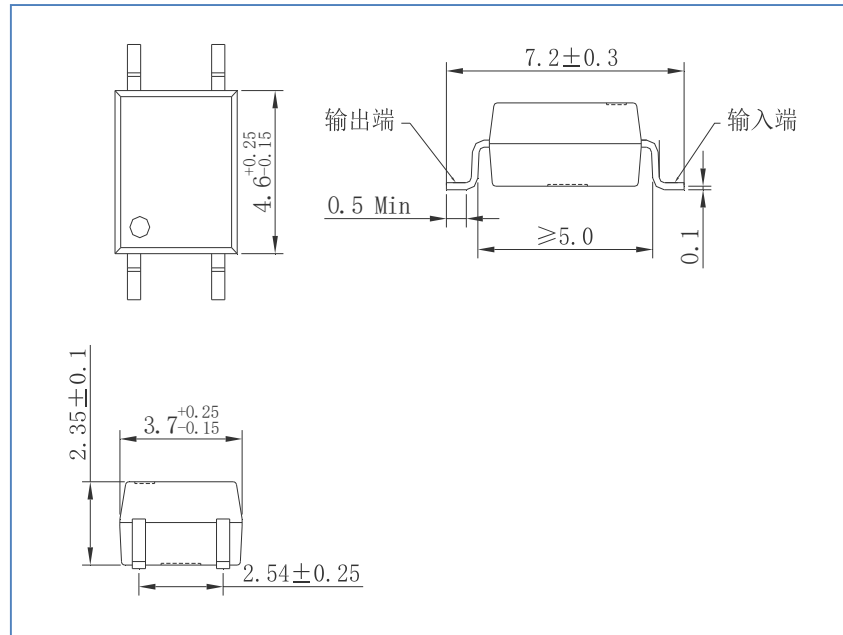
图 4 MT-AQY214S外形尺寸
