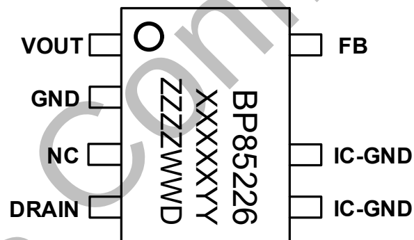
图 3. SOP-7 管脚封装图
