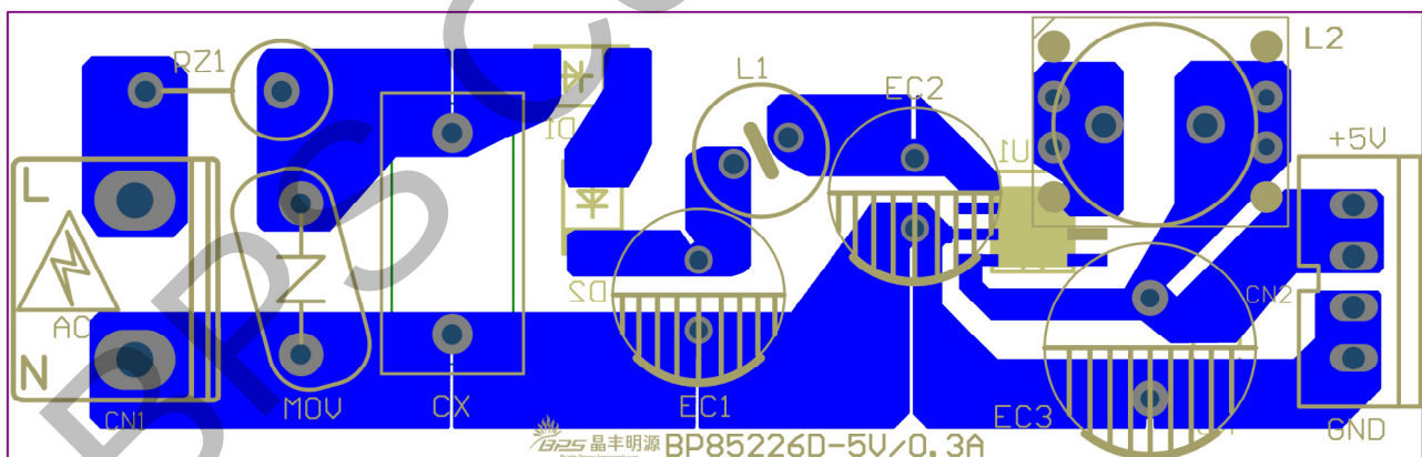
图 14. BP85226D 设计实例 PCB Layout (单面板)
