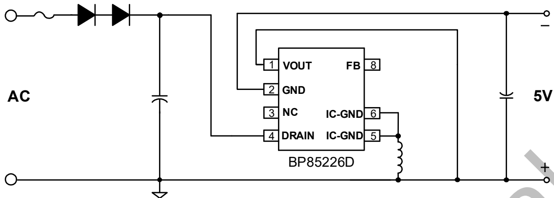
图 2. BP85226D 典型 Buck-Boost 应用电路
