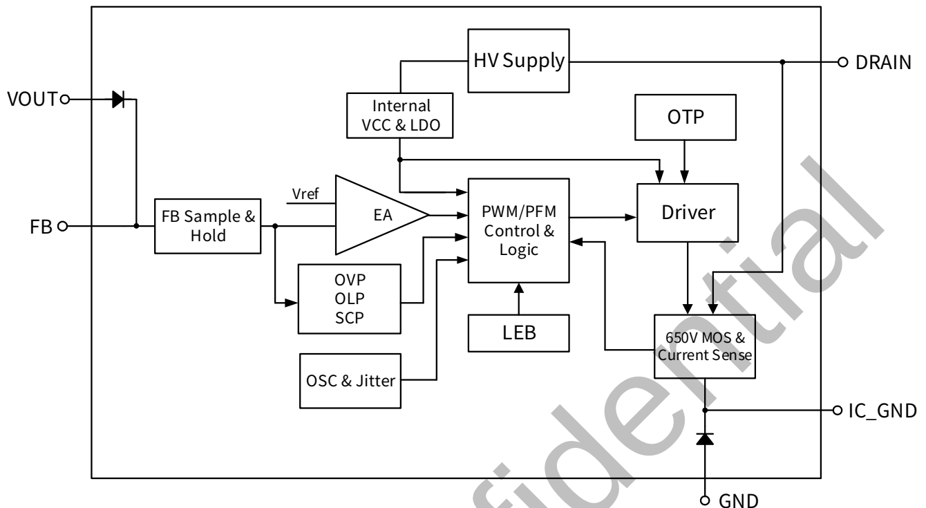
图 4. BP85226D 内部框图
