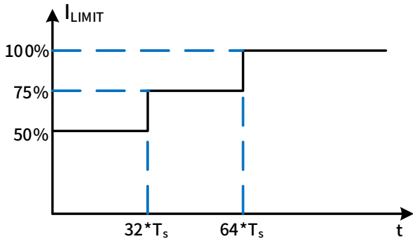
图 6. 软启动过程
