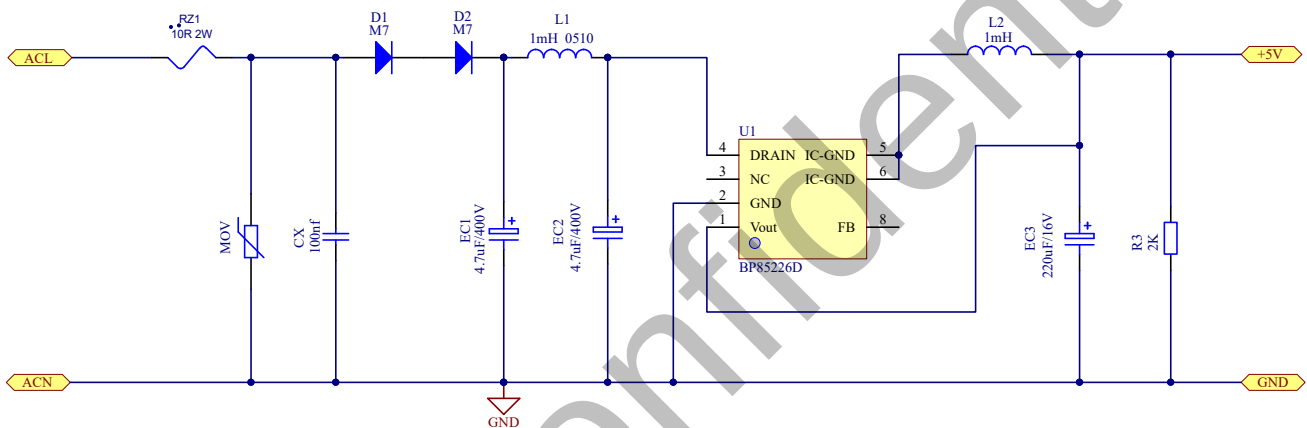
图 13. BP85226D 设计实例电路图，85~265VAC 输入，5V/0.3A 输出
