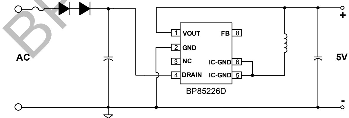
图 1. BP85226D 典型 Buck 应用电路
