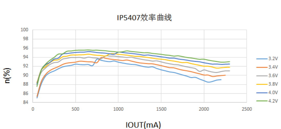
图 4 升压效率曲线图
