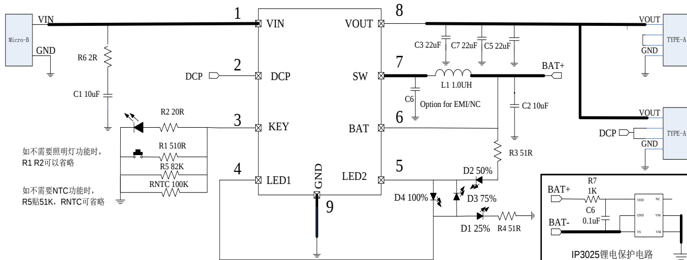
图 7 4LED 电量显示典型应用原理图
